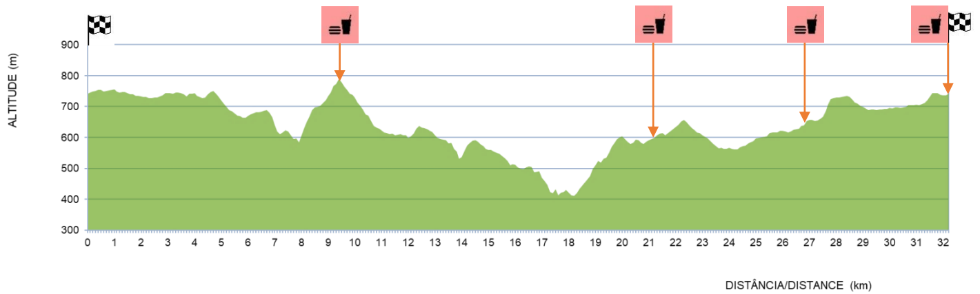
Traçado ADT32K
